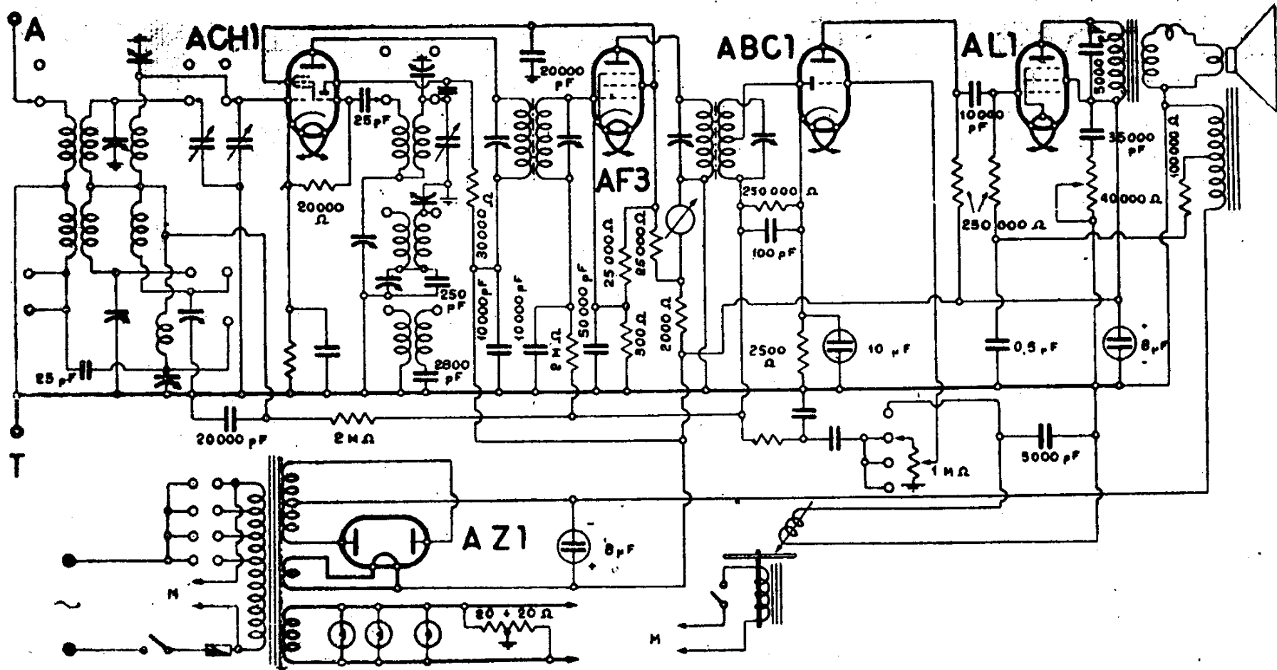
SIEMENS S. A. - MOD. « T 570 FONO »
